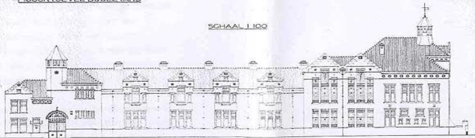
-FIGUUR 2 GEVEL HOOGEN RYNDYK-
