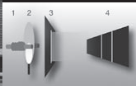
• Illustratie zeemaneffekt.
